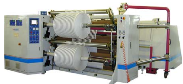
HY-TCB 中心表面分條機 適用各種膠帶分條
