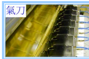
四軸交換分條機 最大捲取直徑: 150mm 最小分條: 12mm
