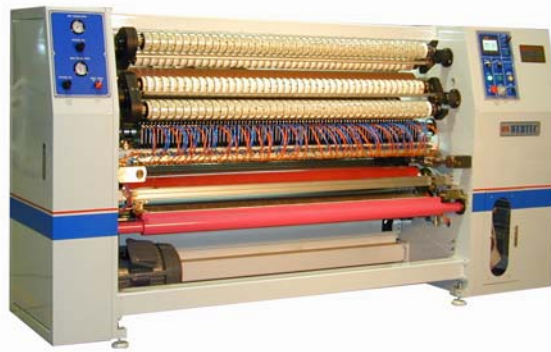
四軸交換分條機 最大捲取直徑: 150mm 最小分條: 12mm
